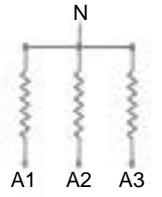
240 : 415 Volt Star Connection
